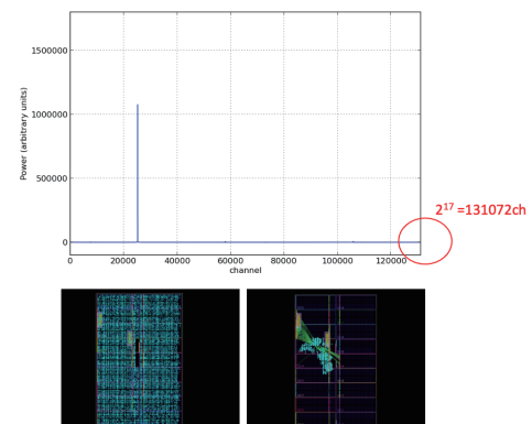
図: (上) 50MHz、-10dBm の信号を入力した時。(下) FPGA 内部のリソース量の比較。左が従来の分光計モデル。右が前積分型分光法モデル。
