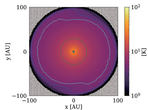
図： \lambda = 1.25mm における等方散乱を考慮した輝度温度 map。コントロールは、3.0K(黒点線)、4.0K(青点線)、5.0K(水色点線)。 a_{min} = 1 \mu m, a_{max} = 1mm, q = 3.5 のダストサイズ分布を仮定。
