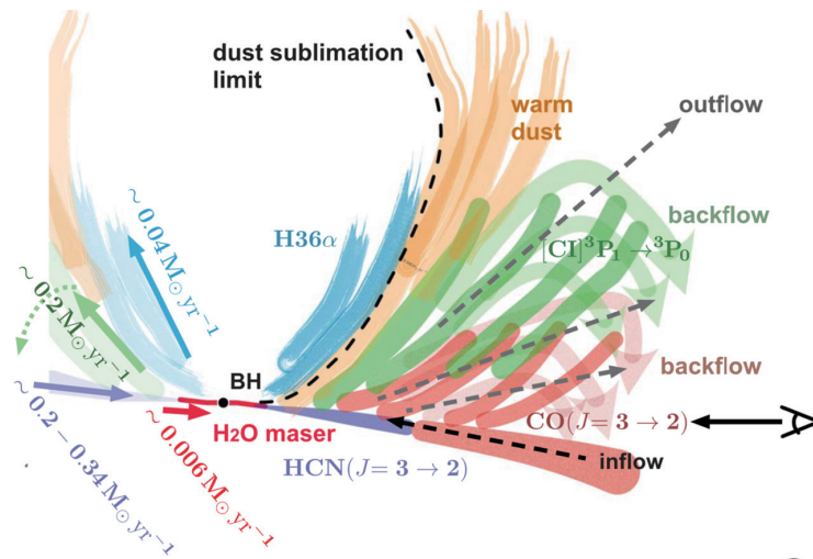
図 2 : 今回の観測結果や他の観測そして理論研究を総合して、Circinus galaxy 中心付近の構造を模式的に示したものです。色の違いはガスの種類（分子や原子、プラズマ）を表す。オレンジ色の部分は暖かい（数 100 K）のダストで、黒点線より内側ではダスト粒子が BH 近傍からの強い輻射を受けて融けてしまう領域。
