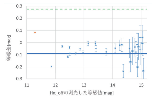
図：VX Cas を含む視野における S/N=10 以上の星の等級差 橙色の点のが VX Cas、青色が VX Cas 以外の星、青色の直線が VX Cas 以外の星の平均値、緑色が 3 シグマを示す。
