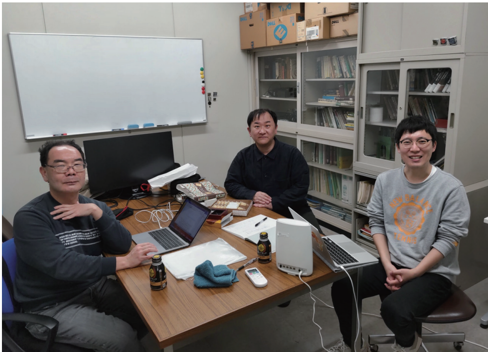
図4: 天の川銀河研究センターに共同研究のために集まった AGN 研究者 (2024 年 2 月撮影)。 右端が筆者のひとり (泉)。左が上田佳宏京都大学教授、中央は長尾愛媛大学教授 (天の川銀河研究センター客員研究員)。それぞれ X 線、光赤外、電波の観測の専門家であり、科学研究費補助金・基盤 A 「活動銀河核構造の全波長域新パラダイムの確立」(研究代表: 和田桂一) のメンバーとして AGN 研究を多角的に進めている。
