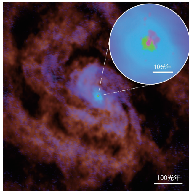
図1: アルマ望遠鏡で観測したコンパス座銀河の中心部。中密度分子ガスを反映する一酸化炭素 (CO) の分布を赤色、原子ガスを反映する炭素原子 (C) の分布を青色、高密度分子ガスを反映するシアン化水素 (HCN) の分布を緑色、プラズマガスを反映する水素再結合線 (H36 \alpha ) の分布をピンク色で示しています。図の中央には活動銀河核が存在します。この銀河は外側から内側に行くにつれて傾いた構造を持つことが知られており、中心部では高密度分子ガス円盤を横から見る形に近づきます。この高密度分子ガス円盤(図の中心部の緑色領域: 右上のズームも参照)の大きさは直径約6光年程度で、アルマ望遠鏡の高い解像度で初めて明確に捉えることができました。プラズマ噴出流は、この高密度分子ガス円盤とほぼ直交する方向に出ています。Credit: ALMA (ESO/NAOJ/NRAO), T. Izumi et al.
