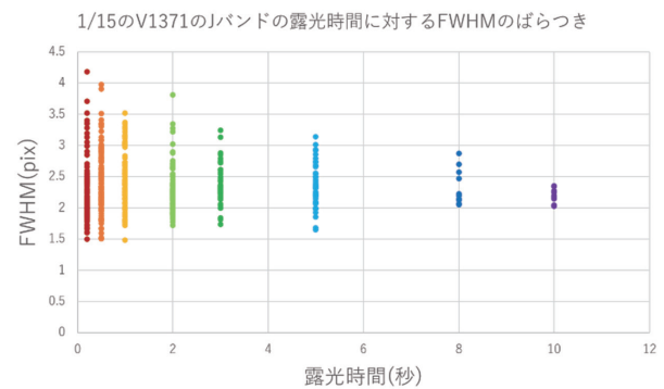
図：露光時間ごとの FWHM のばらつき (Jバンドで撮影) 縦軸は FWHM の大きさ、横軸は露光時間を示す。
