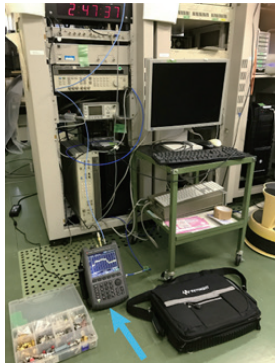
写真1：鹿児島大学の備品となっている携帯スペアナ（水色矢印）とそれを取り巻く VLBI バックエンド機器。2025 年 2 月 17 日野辺山宇宙電波観測所にて撮影。電気回路分析機能（電気信号の透過や反射等を計測する機能）及びベクトル電圧計測機能（2つの交流電気信号間の振幅比及び位相差を計測する機能）も有する。
