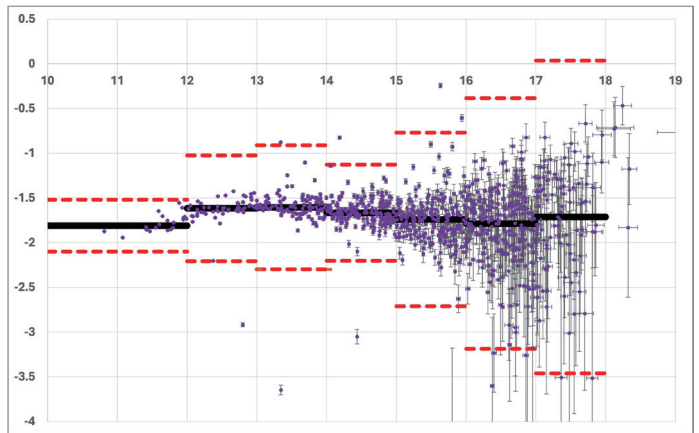
図：横軸は H \alpha _off 等級を Pan-STARRS r 等級として較正した等級、縦軸はそれぞれ等級に直した後の等級差 H \alpha _off 等級 - H \alpha 等級の値を 4 視野分合わせてプロットしたもの。
