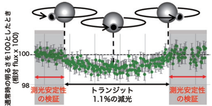
図1: 本研究の検証領域と1m望遠鏡で観測したTOI2154のJバンドライトカーブ。
