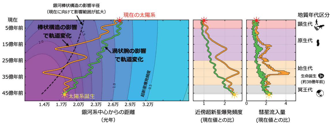
図2：太陽系軌道移動モデルに基づく周辺環境の変動の様子。(左) 2通りの太陽系の軌道半径が時間とともにどのように変化したかを示した図(オレンジ色、緑色の線)。背景の色は銀河系内での超新星爆発頻度の違いを表している。(右) 2つの軌道変化における太陽系周辺の超新星爆発頻度と彗星流入率の時間変化を示した図。太陽系が誕生した過去の時代には周辺で超新星爆発やガンマ線バーストが頻繁に発生しており、銀河系の重力影響による彗星流入率も高かったと予測される。軌道運動の違いにより、太陽系周辺の環境変動のパターンが大きく異なり、それが地球上の生物進化に与える影響も変わることが示されている。
