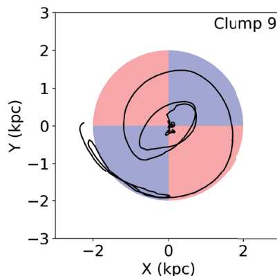
図 2: 棒状ポテンシャルに対するガス塊の軌道。X 軸に棒ポテンシャルを固定しており、第 1、3 象限で減速される。
