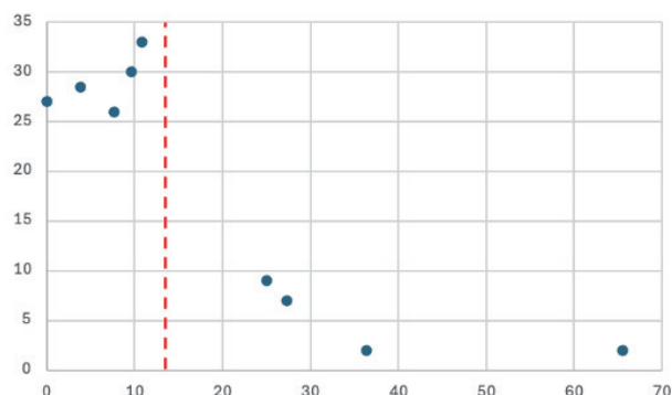
図：温度差とバネの力の相関 横軸：バネの力 (N) 縦軸：温度差 (K) 赤点線：ピンプロブの力
