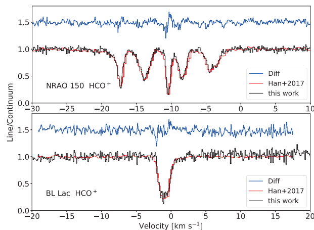
図：背景天体 NRAO 150, BL Lac 方向の 10 年にわたる HCO + 吸収線の強度変動。各スペクトルについて、赤は先行研究 (Han+2017)、黒は本研究、青がそれらの差分を示す。
