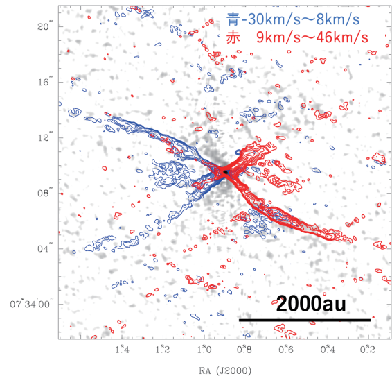
図：B335 から噴き出す ^{12}\text{CO} の積分強度図
