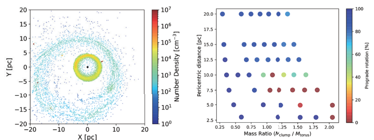
左図：逆回転構造の数密度分布 右図：近点距離と質量比の関係 (カラーバー：順回転の割合)
