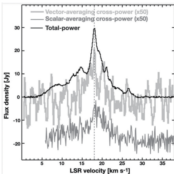
図2: おおいぬ座VY星の一酸化ケイ素(SiO) v=0, J=1 \rightarrow 0 輝線のスペクトル。細い黒線はNRO 45m望遠鏡で取得した全電力スペクトル(スペクトルベースライン差引後)。細い灰色線はメーザー検出を示すクロスパワースペクトルの一例(VERA 入来局-NRO 45m ベースライン、わかりやすくするためスペクトルベースラインをオフセットし、フラックス密度を50倍に拡大表示)。太い灰色線はNRO 45m望遠鏡を含む複数ベースラインの組み合わせによるベクトル平均クロスパワースペクトル。垂直点線は星の視線速度、 V_{\text{LSR}} = 17.9 \text{ km s}^{-1} における ^{28}\text{SiO} v=0 メーザー放射のピーク位置を示す。
