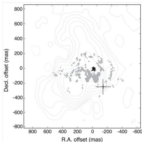
図 1: VY CMa の星周領域における各種メーザーと連続波放射の空間分布。黒の点の塊 (一酸化ケイ素 (SiO) v \geq 1 メーザースポットの位置) のあたりに星が位置している。グレーの等高線は周波数 321 GHz の連続波放射、大きな「+」印は今回、VERA + 野辺山 45m 望遠鏡で検出した SiO v=0, J=1 \rightarrow 0 メーザースポットの位置を表す。シンボルのサイズ (100 ミリ秒角) は最も明るい SiO v=1, J=1 \rightarrow 0 メーザースポットに対する v=0 メーザースポット位置の不確実性に対応する。灰色の小点は水 ( H_2O ) の JK_a, K_c = 10_{2,9}-9_{3,6} 遷移メーザースポットを示す。
