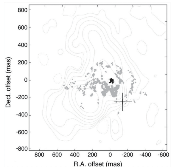
図 1: VY CMa の星周領域における各種メーザーと連続波放射の空間分布。黒の点の塊 (一酸化ケイ素 (SiO) v \geq 1 メーザースポットの位置) のあたりに星が位置している。グレーの等高線は周波数 321 GHz の連続波放射、大きな「+」印は今回、VERA + 野辺山 45m 望遠鏡で検出した SiO v = 0, J = 1 \rightarrow 0 メーザースポットの位置を表す。シンボルのサイズ (100 ミリ秒角) は最も明るい SiO v = 1, J = 1 \rightarrow 0 メーザースポットに対する v = 0 メーザースポット位置の不確か性に対応する。灰色の小点は水 ( H_2O ) の JK_a, K_c = 10_{2,9} - 9_{3,6} 遷移メーザースポットを示す。
