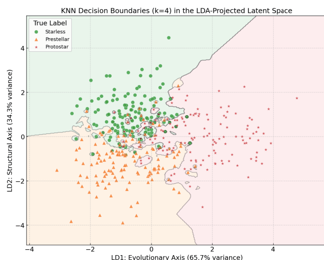
図：VAE で構築した潜在空間 z=64 を線形判別分析により二次元に圧縮した図。 LD1 は進化軸と解釈でき、LD2 は形態的な軸と解釈できる。
