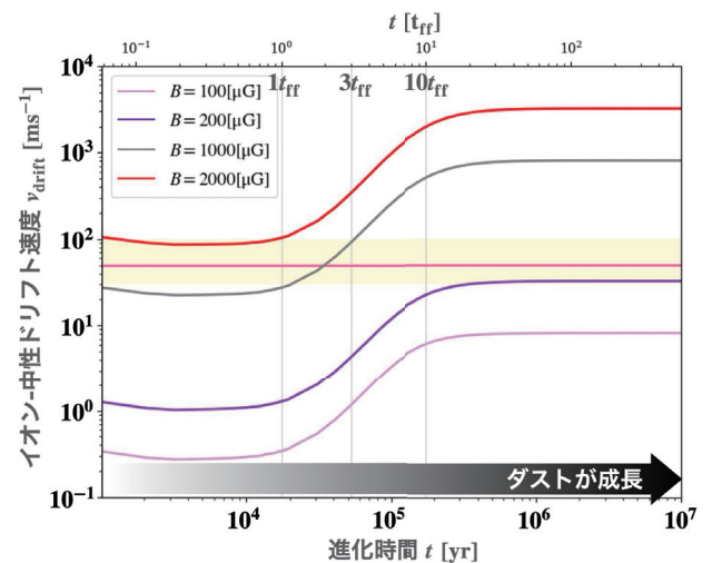
図 1: 推定ドリフト速度進化の磁場強度依存性。横軸は進化時間を示し、ダストの成長に対応する。観測値の範囲を黄色で示す。
