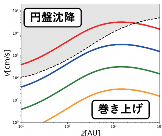
図：ガスの巻き上げ速度 (破線) と重力速度 (実線) の比較
