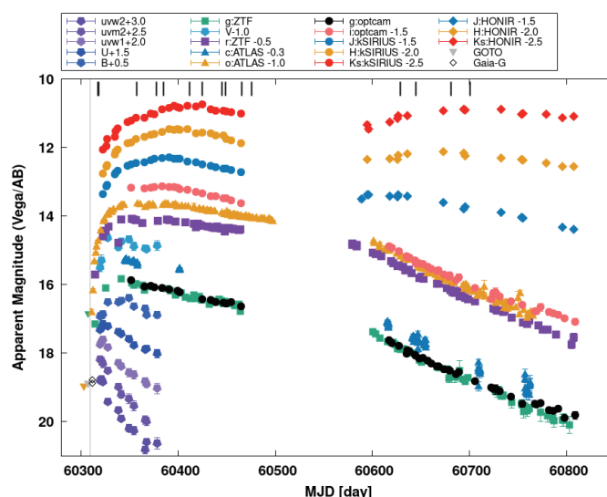
図：SN 2024dyの多バンド光度曲線。横軸は爆発からの時間、縦軸は見かけの等級。近赤外線バンドにおいて、ダスト放射由来の超過が見られる。
