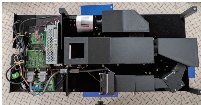
図：開発を行った可視光プリズム分光器の外観
