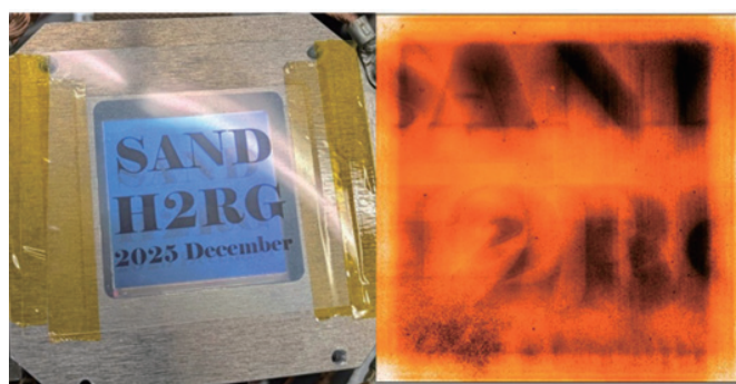
図：検出器に文字の影を映した動作確認画像。右図で暗くなっている部分が文字の影になっている。
