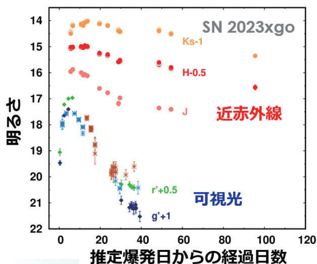
図：kSIRIUS で得られた超新星 SN 2023xgo の光度変化。可視光線では公開されているサーベイ観測によるデータを用いている。可視光で急減光している一方で、近赤外線波長で非常な緩やかな変化だったことがわかる
