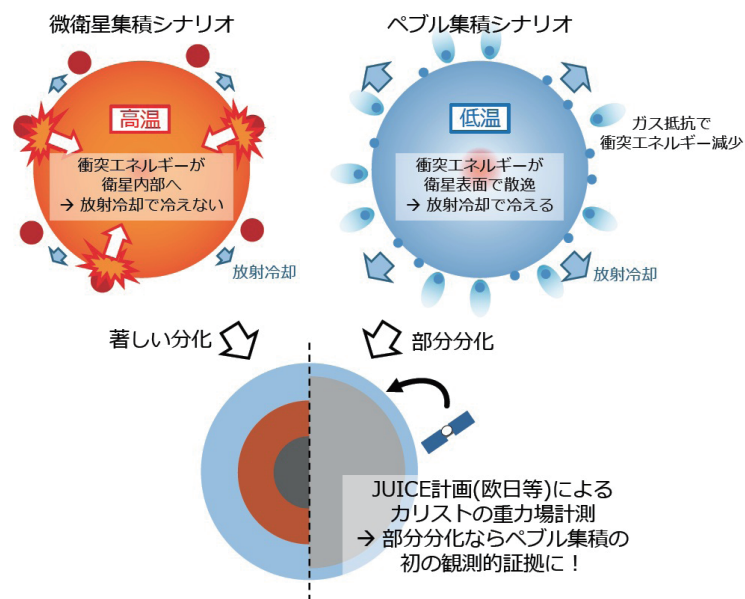
図 2：微衛星集積シナリオとペブル集積シナリオにおけるカリスト内部の概念図。微衛星集積シナリオでは、衛星内部に衝突エネルギーが伝わり衛星が高温になるが、ペブル集積シナリオでは、衝突エネルギーが衛星表面で散逸し、放射冷却により衛星内部が低温に保たれる。また、ペブルはガス抵抗を受けやすく、衝突エネルギーが減少する。結果として、微衛星集積では内部が著しく分化し、ペブル集積では部分的にしか分化しない。もし JUICE 計画によるカリストの重力場観測により部分分化が確認できれば、ペブル集積の初の観測的証拠になりうる。
