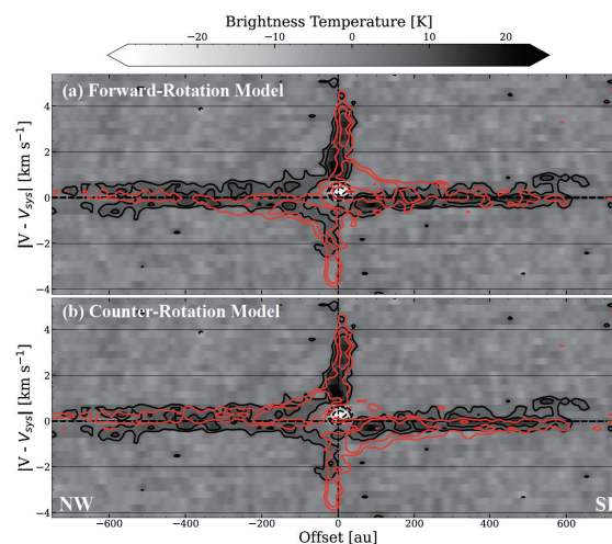
図：長軸に沿った \text{H}^{13}\text{CO}^+(4-3) 輝線の、観測データ (黒色 contour + グレースケール) とモデルデータ (赤色 contour) による PV 図の比較。パネル(a)は、円盤とエンベロープが同じ方向に回転しているモデル、パネル(b)は逆回転 (counter-rotating) しているモデルの PV 図を示す。contour レベルは -20, -10, -5, -3, 3, 5, 10, 20 \sigma ( 1\sigma = 2.5 \text{ mJy beam}^{-1} )。中央の横破線は天体系の静止速度 ( V_{\text{sys}} = 6.12 \text{ km s}^{-1} ) を示し、縦破線は中心星位置を示す。
