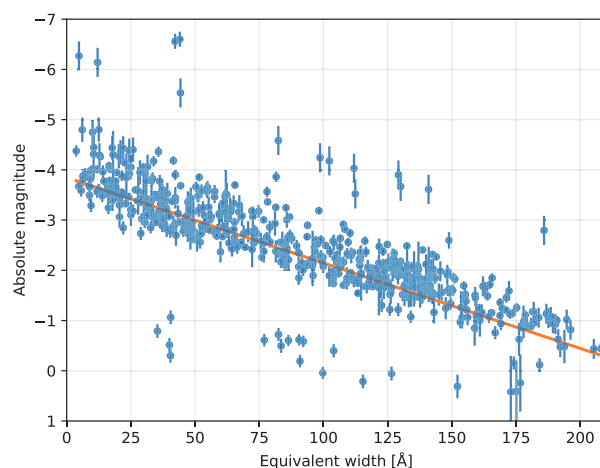
図：全天体における Ic バンド絶対等級と VO 吸収線 (1.05 \mu\text{m} ) 等価幅の関係。横軸に等価幅、縦軸に Gaia および VERA の年周視差から算出した絶対等級を示す。
