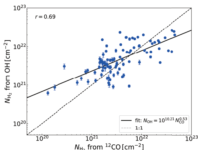
図：CO から推定した \text{H}_2 柱密度 N_{\text{H}_2} と OH から推定した \text{H}_2 柱密度 N_{\text{H}_2} の相関図。実線は両者のべき乗フィットを示し、破線は 1:1 の関係を示す。両者の相関係数は r=0.69 である。
