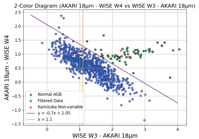
図：[AKARI18 \mu m -WISE All-Sky W4(22 \mu m )]vs[W3(12 \mu m )-AKARI18 \mu m ]の 2 色図。
