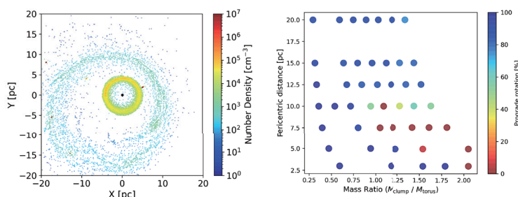
左図：逆回転構造の数密度分布 右図：近点距離と質量比の関係 (カラーバー：順回転の割合)
